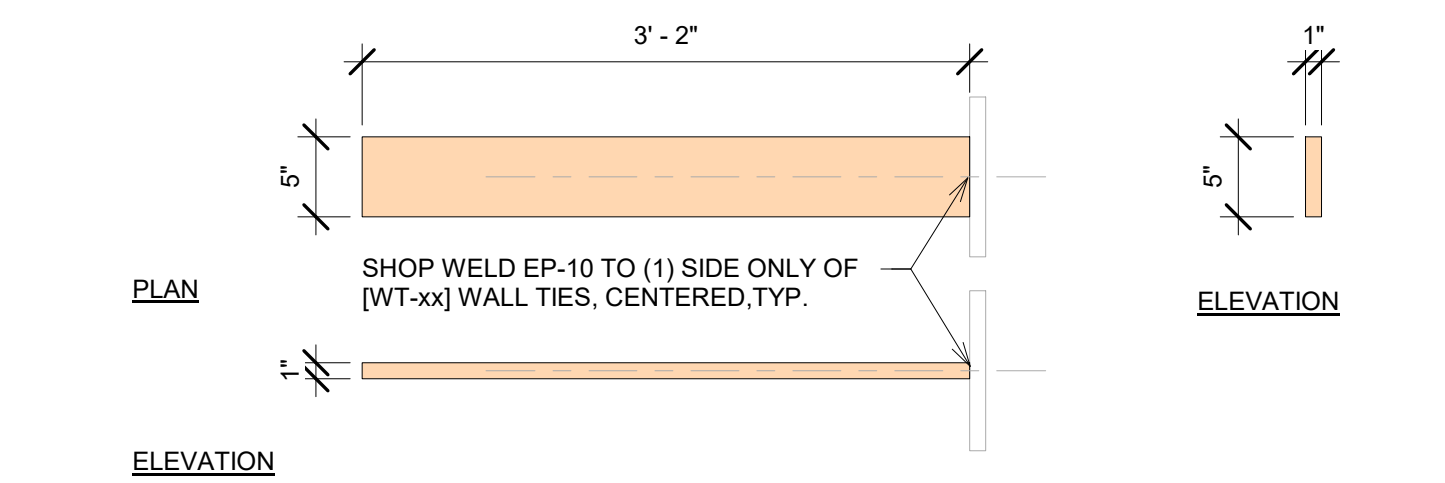
[EP-10] 1" END PLATE SCALE: 1" = 1'-0"
